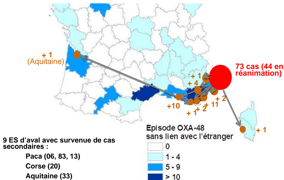
Figure 1. Synthèse des cas d'EPC OXA-48 liés à l'épisode des Alpes Maritimes (N=106) : transfert des patients et cas secondaires dans les établissements d'aval, nombre d'épisodes impliquant des EPC OXA-48 sans lien avec l'étranger, 2004 – 2013, InVS-Raisin / CCLin Sud-Est, 6 janvier 2014.
